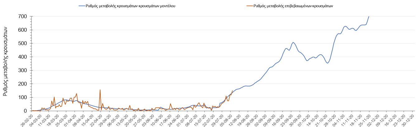
Σχήμα . Ημερήσιος ρυθμός μεταβολής των επιβεβαιωμένων κρουσμάτων και των κρουσμάτων σύμφωνα με την πρόβλεψη του μοντέλου (νέα κρούσματα/ημέρα) μέχρι το τέλος του έτους 2020
